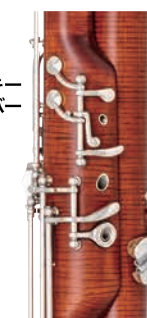
左手キーレイアウト
